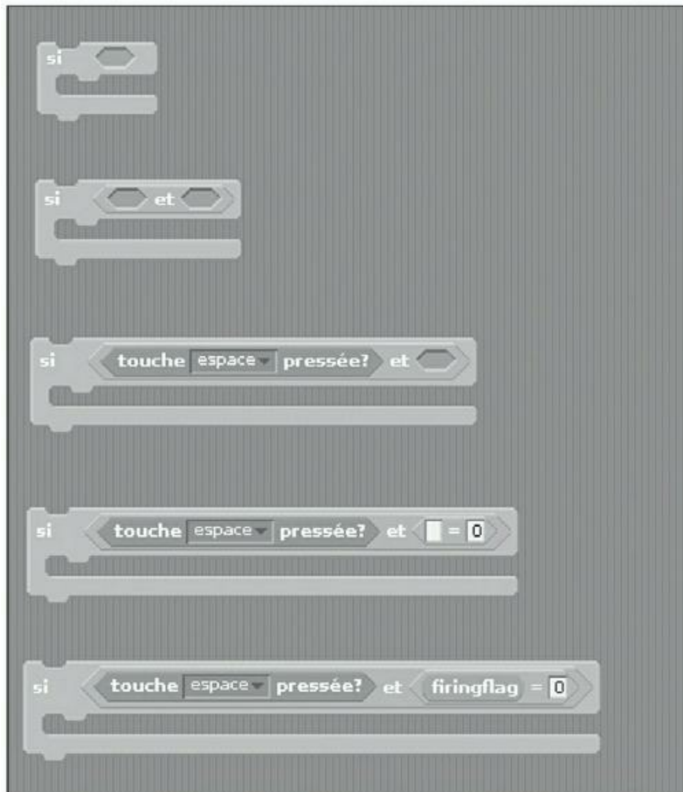
Figure 10.13 : Les différentes étapes de construction d'un bloc conditionnel utilisant deux conditions.
