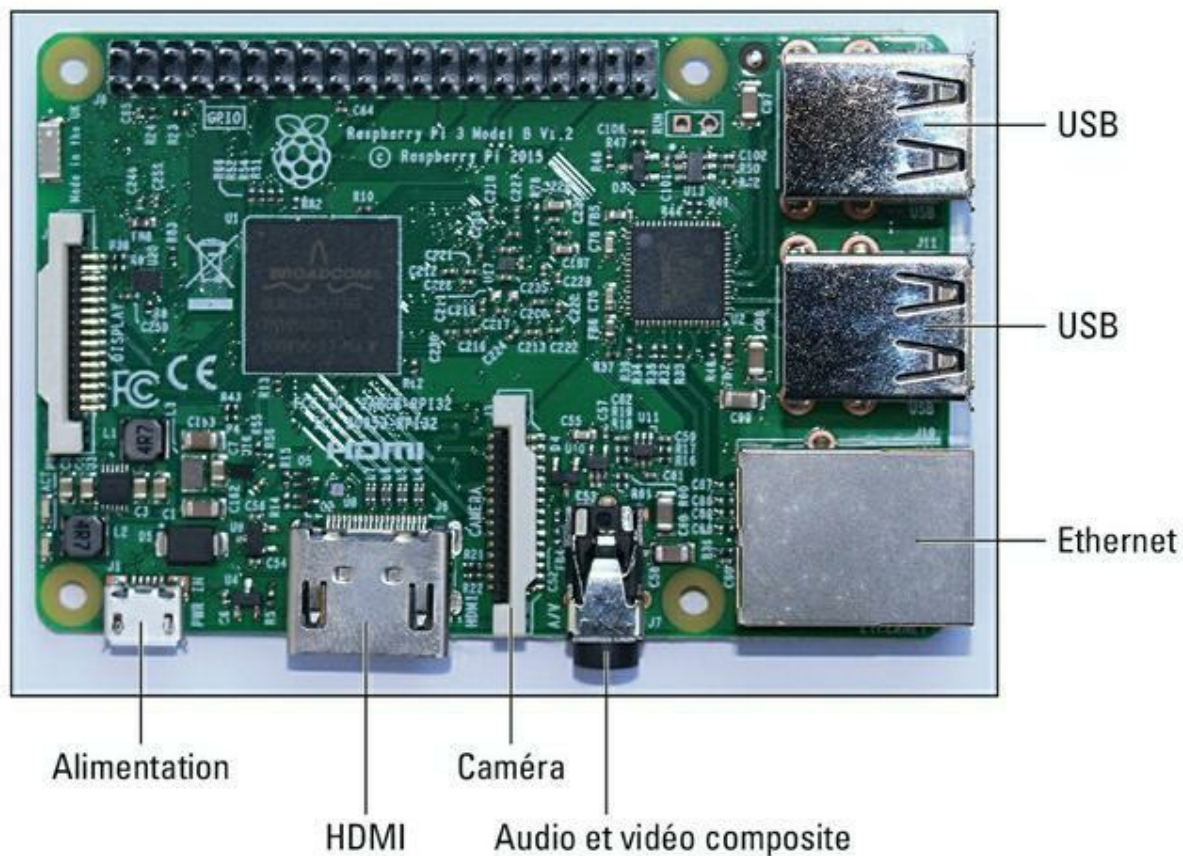
Figure 3.2 : Connexions de la Raspberry Pi 3 et B (valable aussi pour le Pi 2, le modèle B et le modèle A+).
