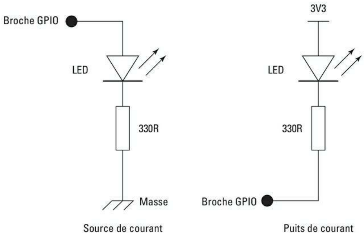
Figure 15.8 : Les deux techniques de pilotage d'une charge LED.
