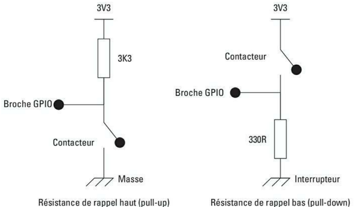
Figure 15.9 : Résistances de rappel haut et bas pour stabiliser une broche d'entrée GPIO.
