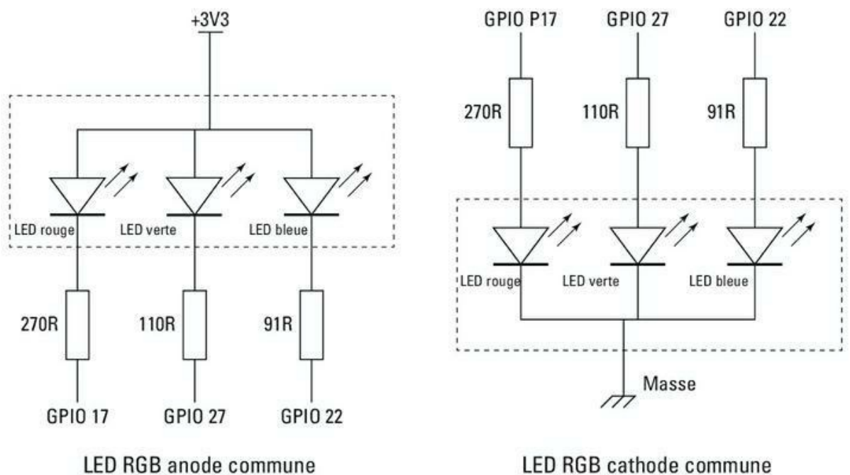
Figure 17.2 : Câblage d'une LED RGB à anode et à cathode commune.
