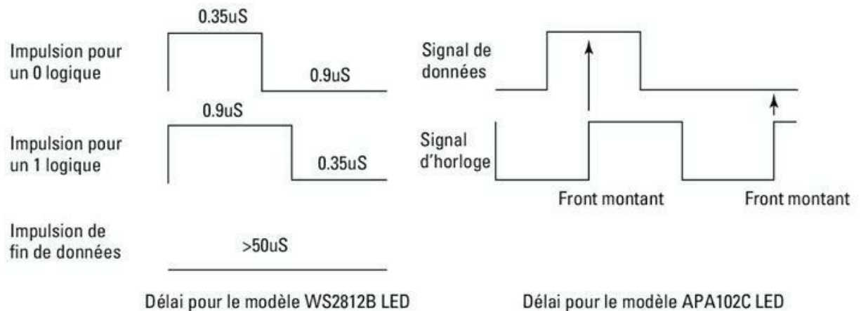
Figure 17.6 : Chronogrammes pour les LED WS2812b et APA102.
